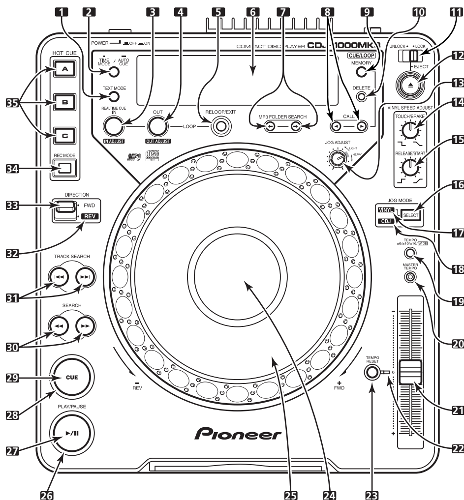
Frontplatte/Pannello anteriore
