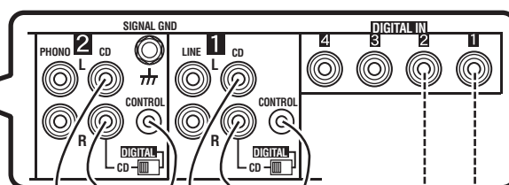
Esempio di collegamenti DJM-800:
