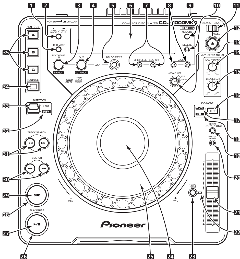
Voorpaneel/Panel frontal
