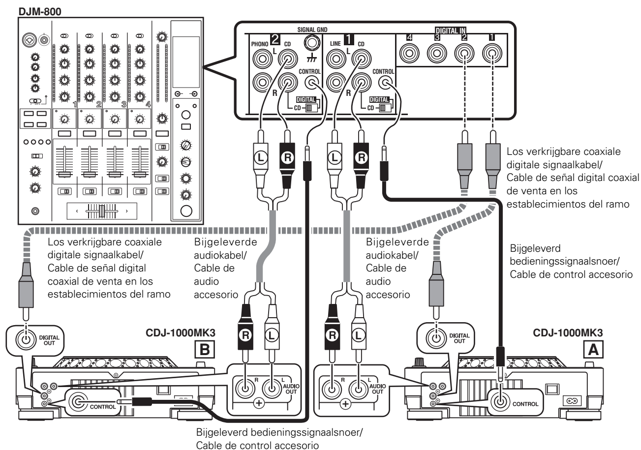
Ejemplo de conexión del DJM-800:
