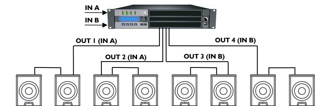
Figure 6 : 8 enceintes 8XT connectées à un contrôleur LA4 / LA4X
