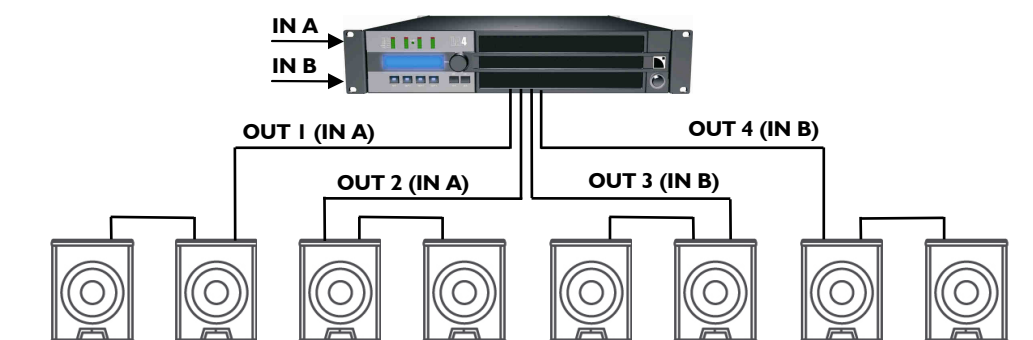
Figure 5 : Huit enceintes 8XT connectées à un contrôleur LA4 / LA4X
