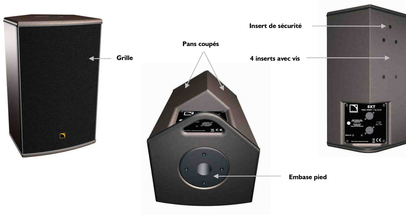
Figure 3 : L'enceinte 8XT
