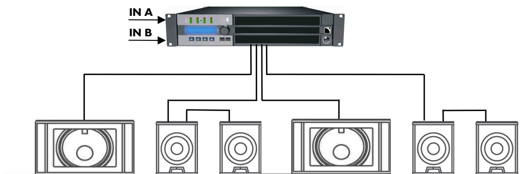
Figure 7 : Quatre 8XT et deux SB18 connectées à un contrôleur amplifié LA4 / LA4X
