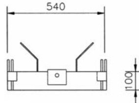
Type DPA ..... Raccord bac à chaîne
