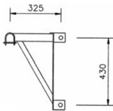
Type A1D M/F ..... Angle linéaire M/F
